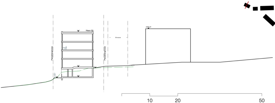
Richtprojekt Schönegg: Schnitt F - F
