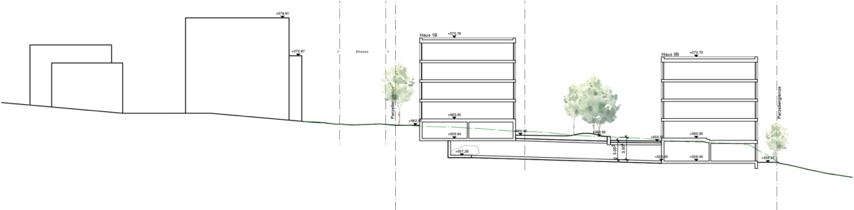
Richtprojekt Schönegg: Schnitt B - B
