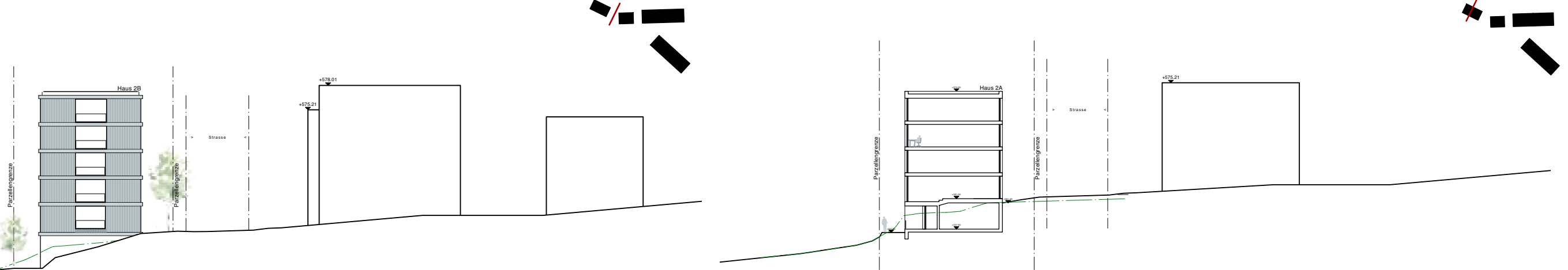
Schnitt F - F 1 - 500
